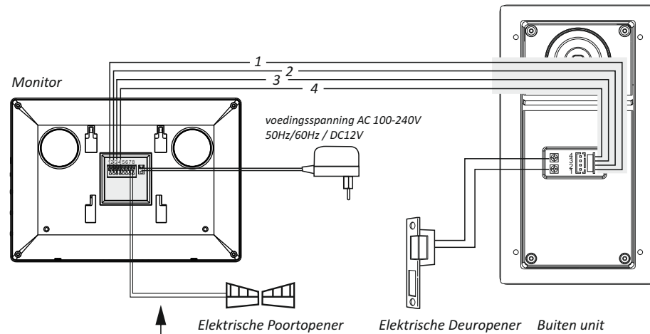
Bedradingsdiagram elektrische deur ontgrendeling (verbonden met outdoor unit)
