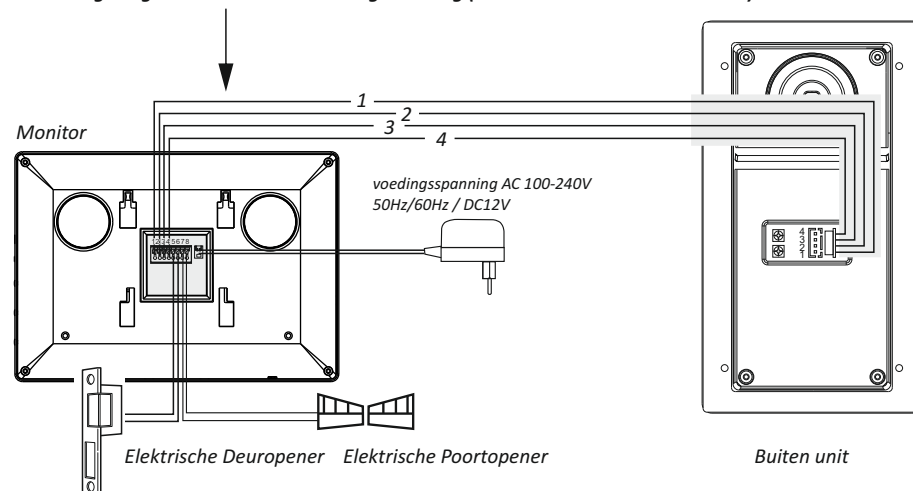
Bedradingsdiagram elektrische deur ontgrendeling (verbonden met indoor monitor)
