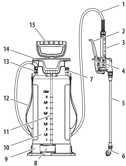
Teile des Drucksprüngeräts
